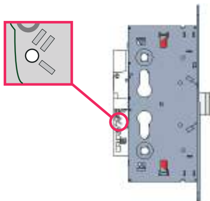
Figura 2: foro per la temporizzazione
