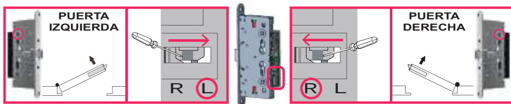
Figura 1: palanca para cambio de “mano”
