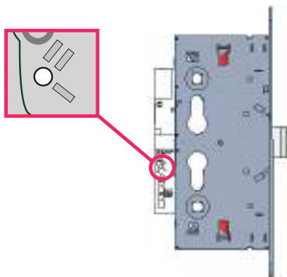
Figura 2: orificio de temporización
